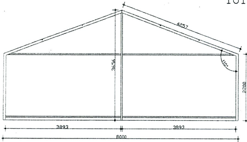
vooraanzicht constructie
