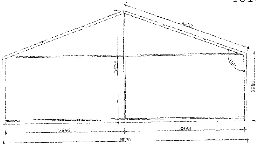
vooraanzicht constructie
